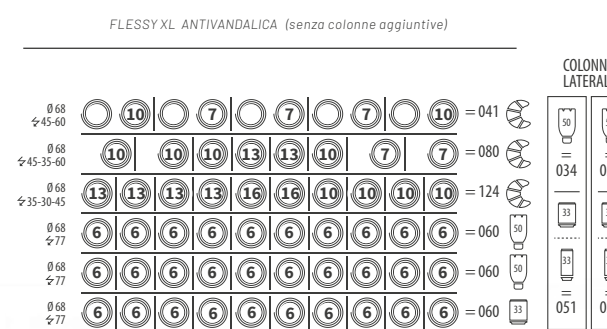
FLESSY XL PLUS ANTIVANDALICA (con colonne aggiuntive)
