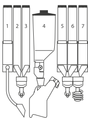
CAFÈ EM GRÃO (configuração válida para versão com grupo de café expresso tradicional + versão com grupo de câmara variável)
